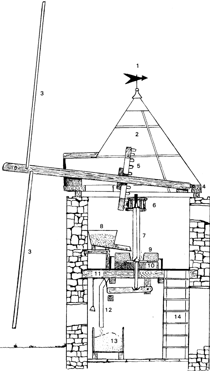
COUPE SCHEMATIQUE D'UN MOULIN A VENT PROVENÇAL
