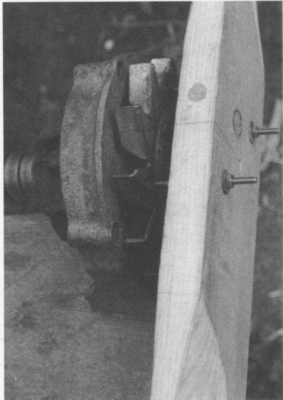
Repeller mit verschiebbar angeschraubter Riemenscheibe zum Prüfen auf die vordere Hälfte der LiMa gesteckt.
