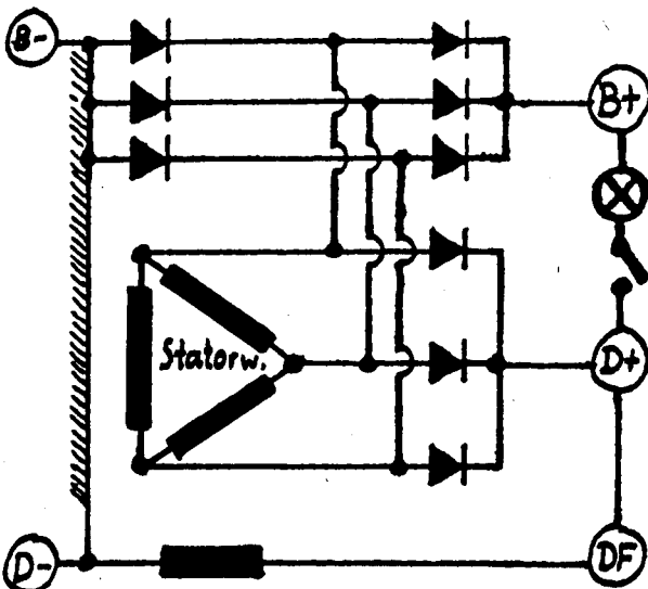
C: wie B, jedoch Dreieckschaltung
