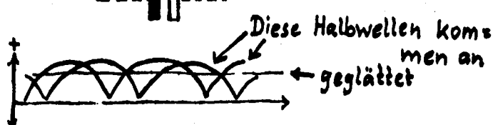
Verminderte Feldspannung durch Brückengleichrichter zwischen 2 Phasen.
