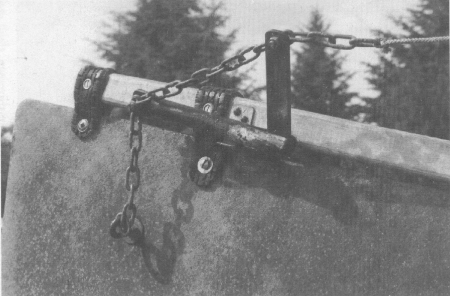
Edel-Bremse (Gesamtbild S. 3): Der Winkelhebel, aus Rohr, Flacheisen, Kette. Die Achse sitzt schräg, damit er die Steuerfahne auch hochziehen kann!
