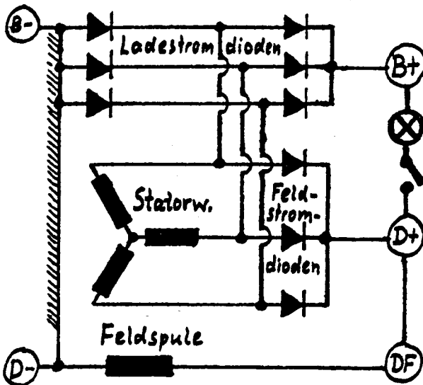
B: Drehstromlima, Sternschaltung, 3 Dioden extra für den Feldstrom (z.B. Bosch 14V 35A, 45A, 55A u.a.)
