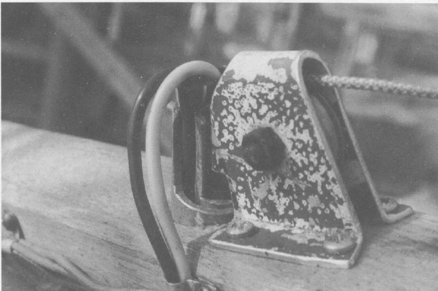
Kabel-/Schlauchbefestigung, daneben Seilrolle im Führungsblech.
