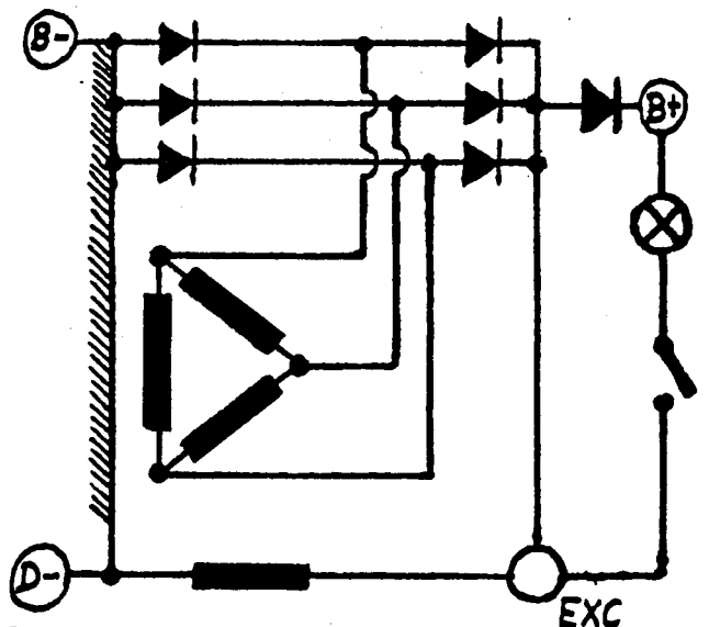
E: wie D, jedoch Dreieckschaltung
