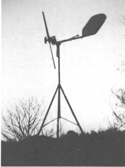
Windrad mit Helikoptersicherung in Betriebsstellung. Gewicht abgehängt - schon halb in Sturmstellung
