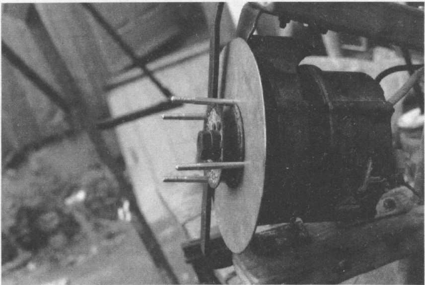
Bremse: Flacheisen drückt gegen die große Blech-Scheibe
