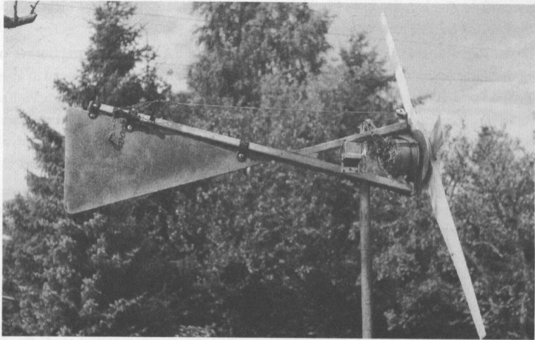
Ein Windrad in der „Standard-Bauweise“ seit 1994 (S.24), mit „Edel-Bremsmechanik“ (S.59)
