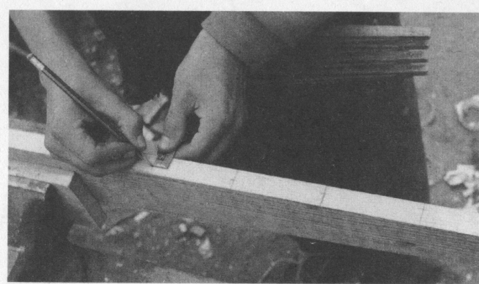
Hinterkanten-Linie: Kontrollpunkte anzeichnen
