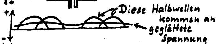
Verminderte Feldspannung durch Einweg-Gleichrichter aus 2 Phasen.
