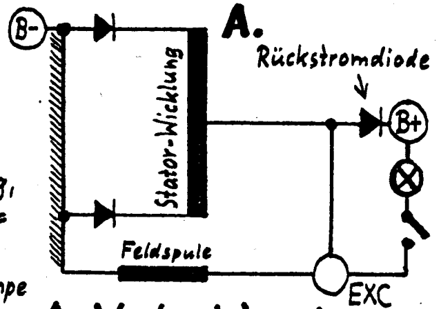
A: Wechselstromlima in Gegentaktschaltung mit Rückstrom-Diode (2 CV).
