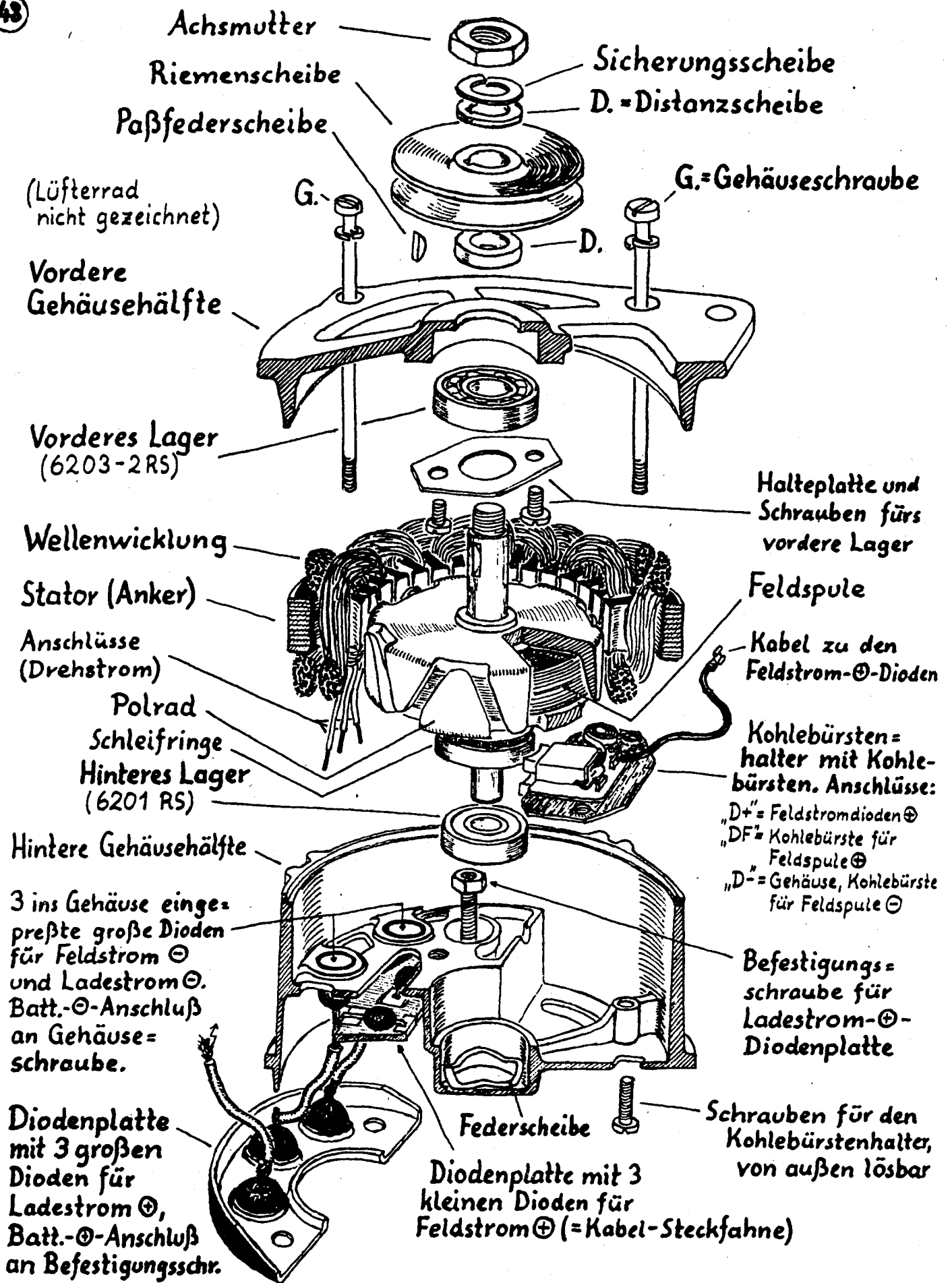
Explosionszeichnung einer Drehstrom-LiMa: Bosch, ältere Bauart mit innen montiertem Kohlebürstenhalter
