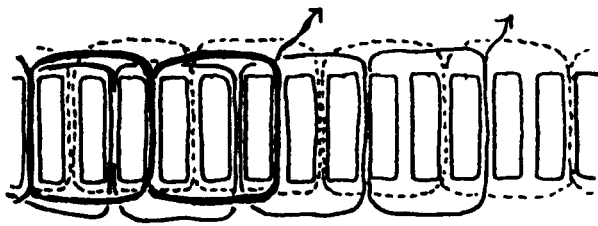
"Dreilagengewicklung", z.B. Original Ducellier u.a.
