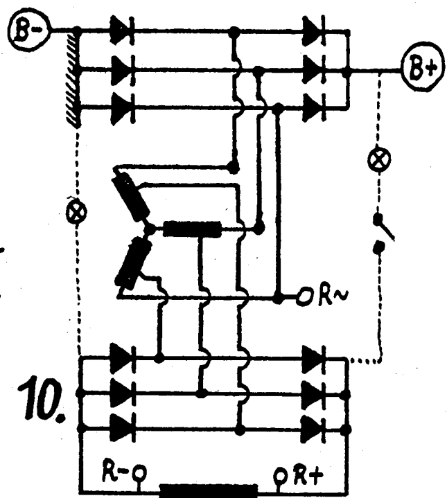
Verminderte Feldspannung aus Anzapfungen an den Wicklungen über Voll-Brückengleichrichter.
