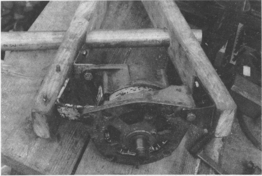
Befestigung der LiMa mit Eisenwinkeln im Dreiecksrahmen
