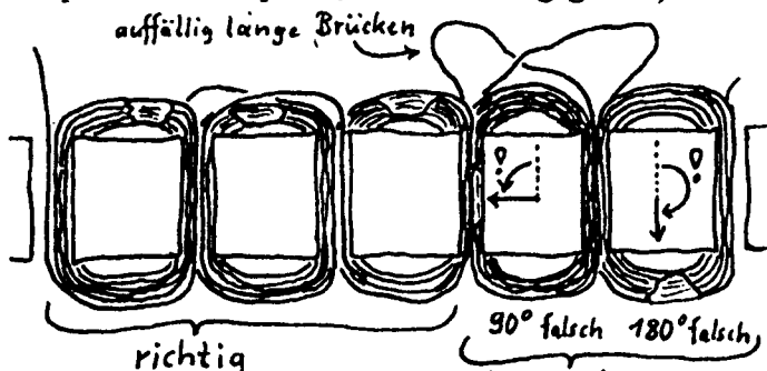
Lage der Spulen. Der Einfachheit wegen nur 1 Strang betrachtet.
