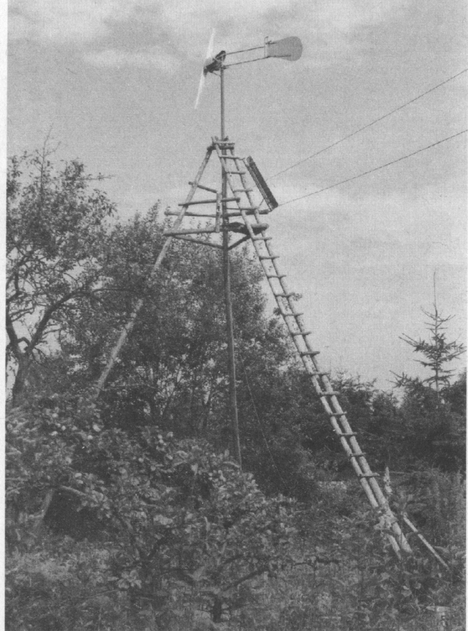
Ein hoher Mast aus 3 dünnen Baumstämmen, stabil und einfach zu bauen, bringt das Windrad aus dem Windschatten.
