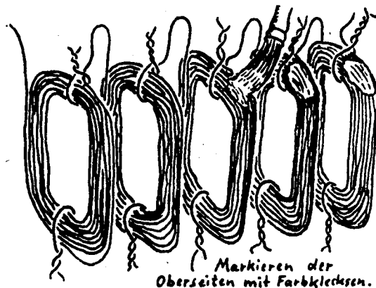
Lage der Spulen. Der Einfachheit wegen nur 1 Strang betrachtet.
