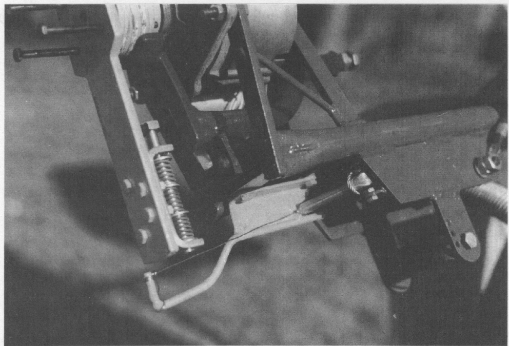
Die Sicherung: Eisen mit Fliehwicht, Haken, Kupferdraht, Seil-Aufhängung.
