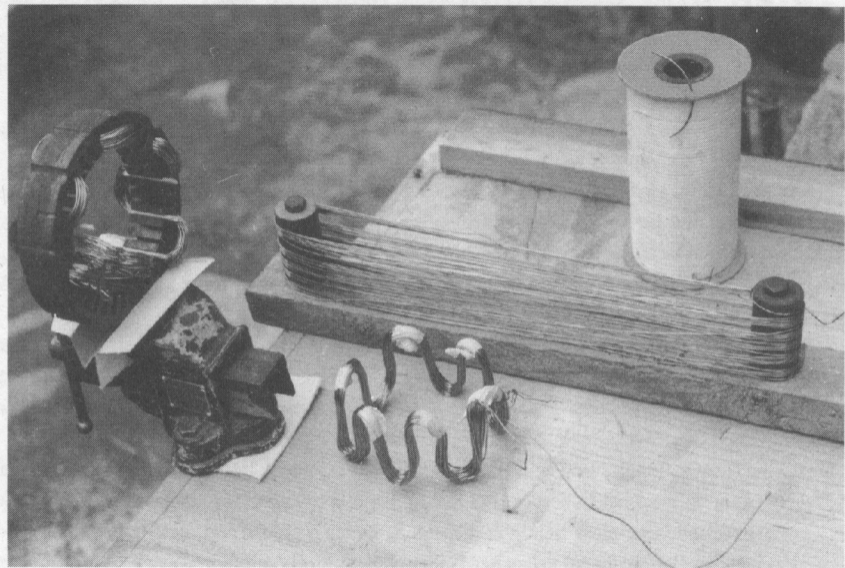
1. Strang fast eingelegt, 2. Strang gebogen, 3. auf der Schablone.
