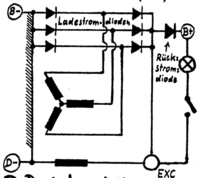
D: Drehstromlima, Sternschaltung, Feldstrom über Ladestromdioden, Rückstromdiode (viele französ. LiMas)
