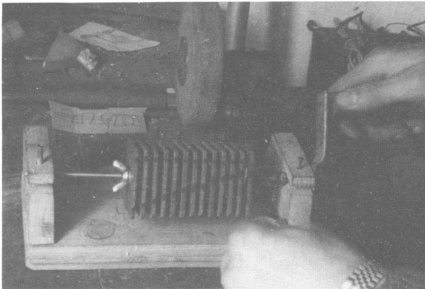
Gebrauch der selbstgebauten Wickelvorrichtung.
