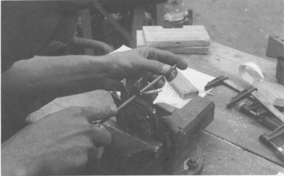
Blech - Riemenscheibe: Aussparungen für Schrauben genau passend zu den Bohrungen im Verstärkungsblech (hier: Lüfterrad) feilen.
