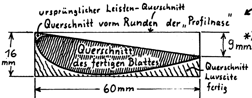
Maßzeichnungen 1:1 zum Abpeusen.
