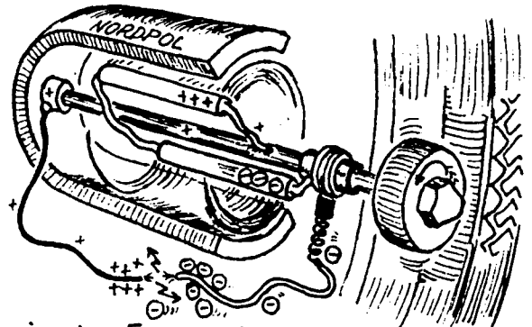
Prinzip des Fahrraddynamos.
