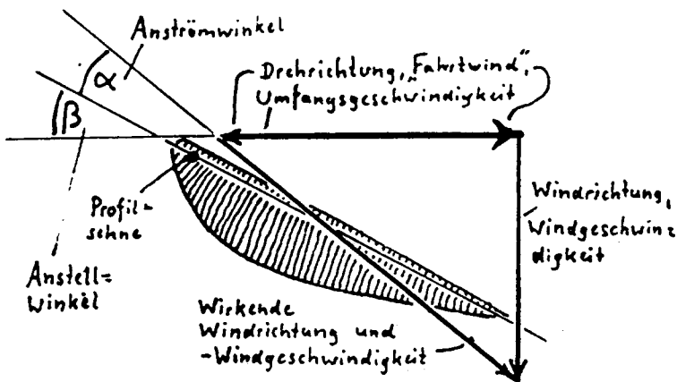
Langsamlaufender Repeller.
