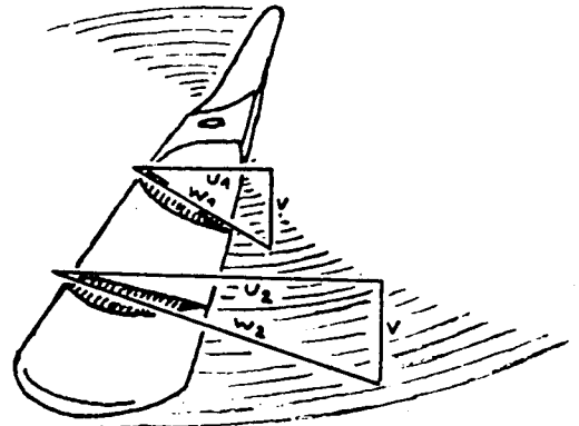
Verwindung des Repellerblattes:
