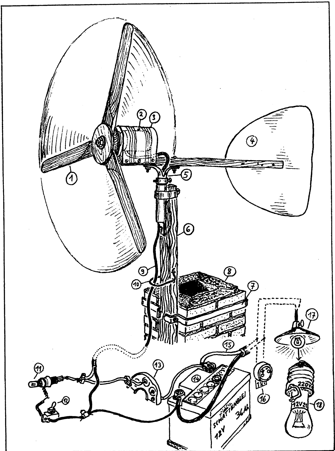
Leistungsfähiges Kleinst-Windrad mit Auto-Gebläse-motor, 80 cm-bis 1m-Repeller und umgewickeltem Anker.
