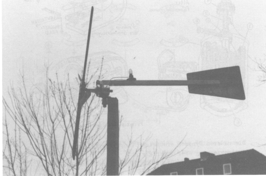
Ansicht des ganzen Dynamowindrades
