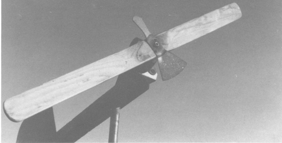
2-Blatt-Repeller, 1 m \phi und Anlaufhilfe eines Gebläsemotor-Windrades.
