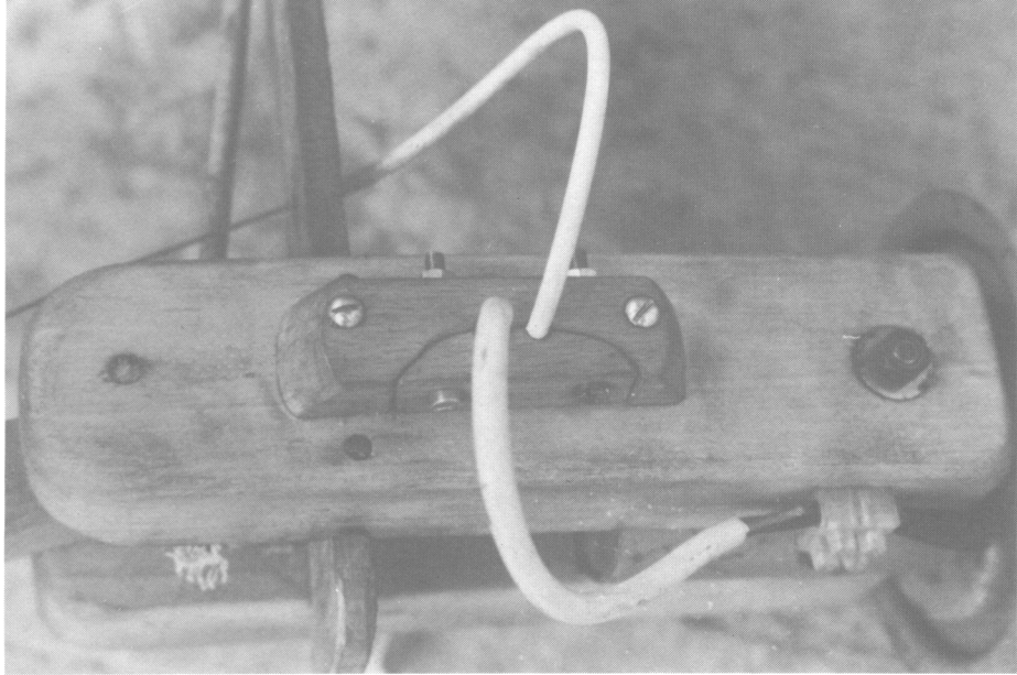
Interessantes Einzelteil: Bowdenzughülle und Kabel müssen gut festgehalten werden. Hier mit einem passend gebohrten und gesägtem Hartholzklötzchen.
