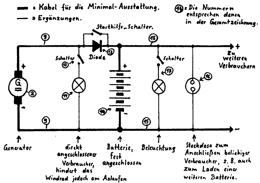
Schaltplan der Windstrom-Anlage.
