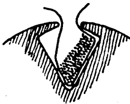
Erster Isolierstreifen eingelegt, erste Wicklung in der Nut.
