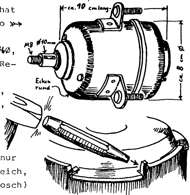
Genietetes Gehäuse.
