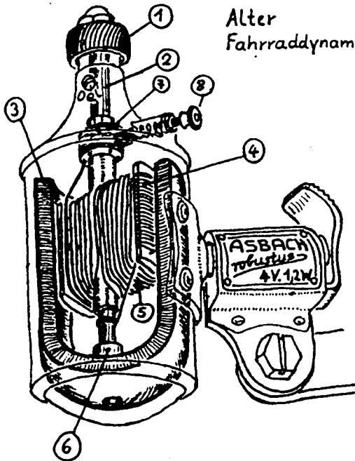
Prinzip des Fahrraddynamos.
