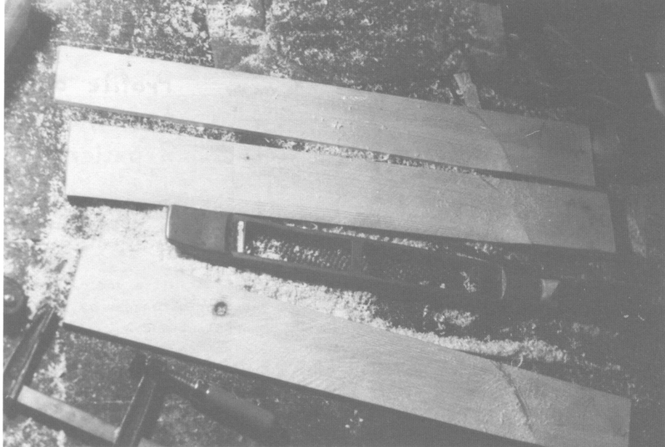
Bearbeiten der Luvseite: unten-geraspelt, Mitte-gefeilt, oben-trapezförmig gehobelt
