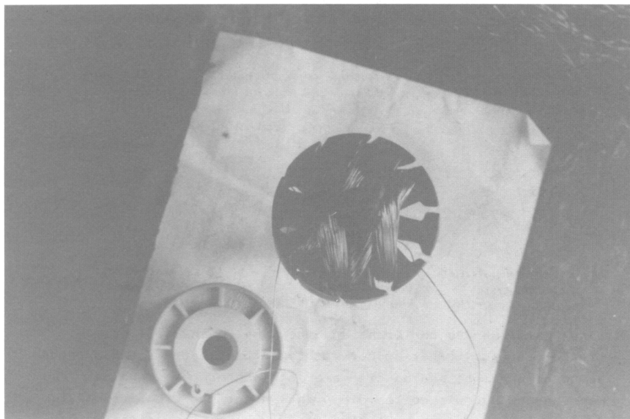
10-poliger Anker, 2 Spulenpaare fertig gewickelt.
