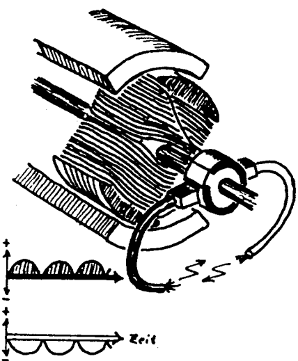
Gleichstrom-Generator hat einen Kommutator mit Lamellen
