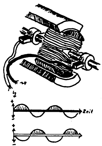
Wechselstrom-Generator (alter Fahrraddynamo) hat Schleifringe
