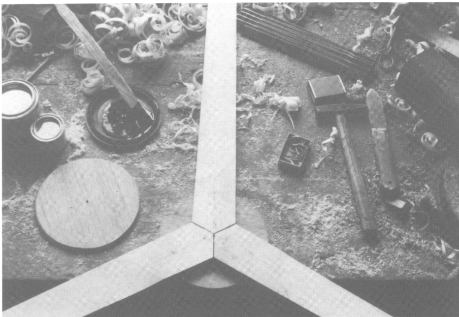
Zusammenleimen der vorgearbeiteten Blätter.
