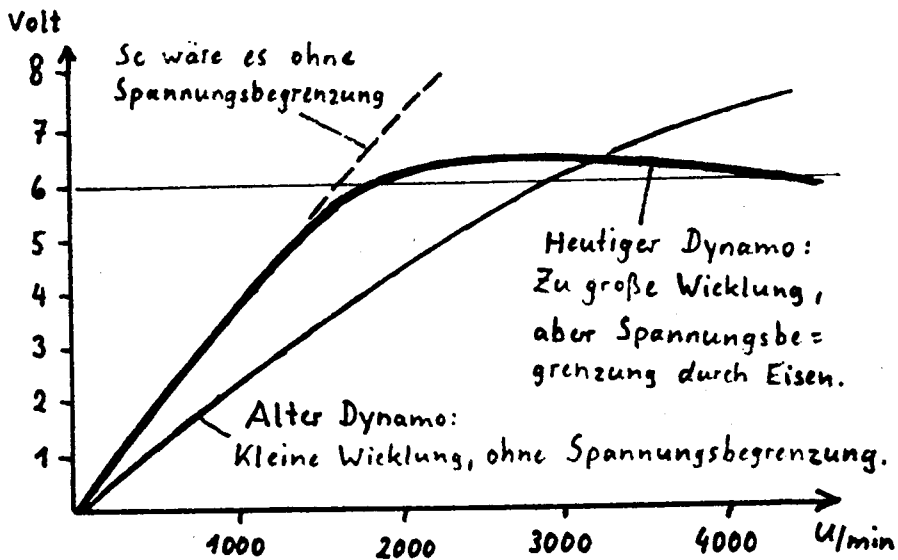
Ungefähre Kennlinien von Dynamos.
