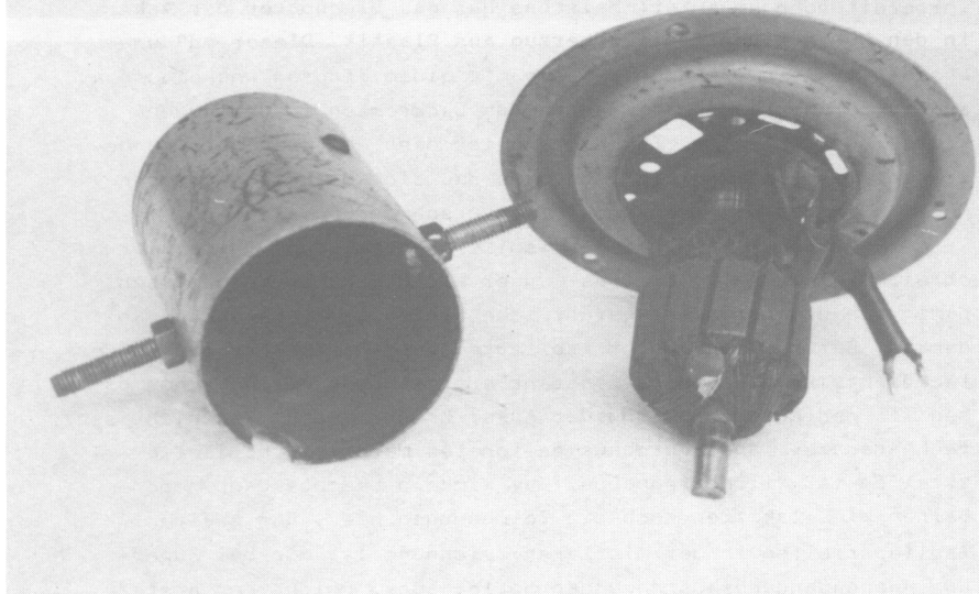
Ein Auto-Heizungs-Gebläsemotor, aufgeschraubt. Links das Gehäuse mit 2 Dauermagneten. Die Schrauben sind selbst hineingebastelt zur Befestigung am Rahmen. Rechts der Anker, Kommutator, Kohlebürstenhalter, Gehäusedeckel
