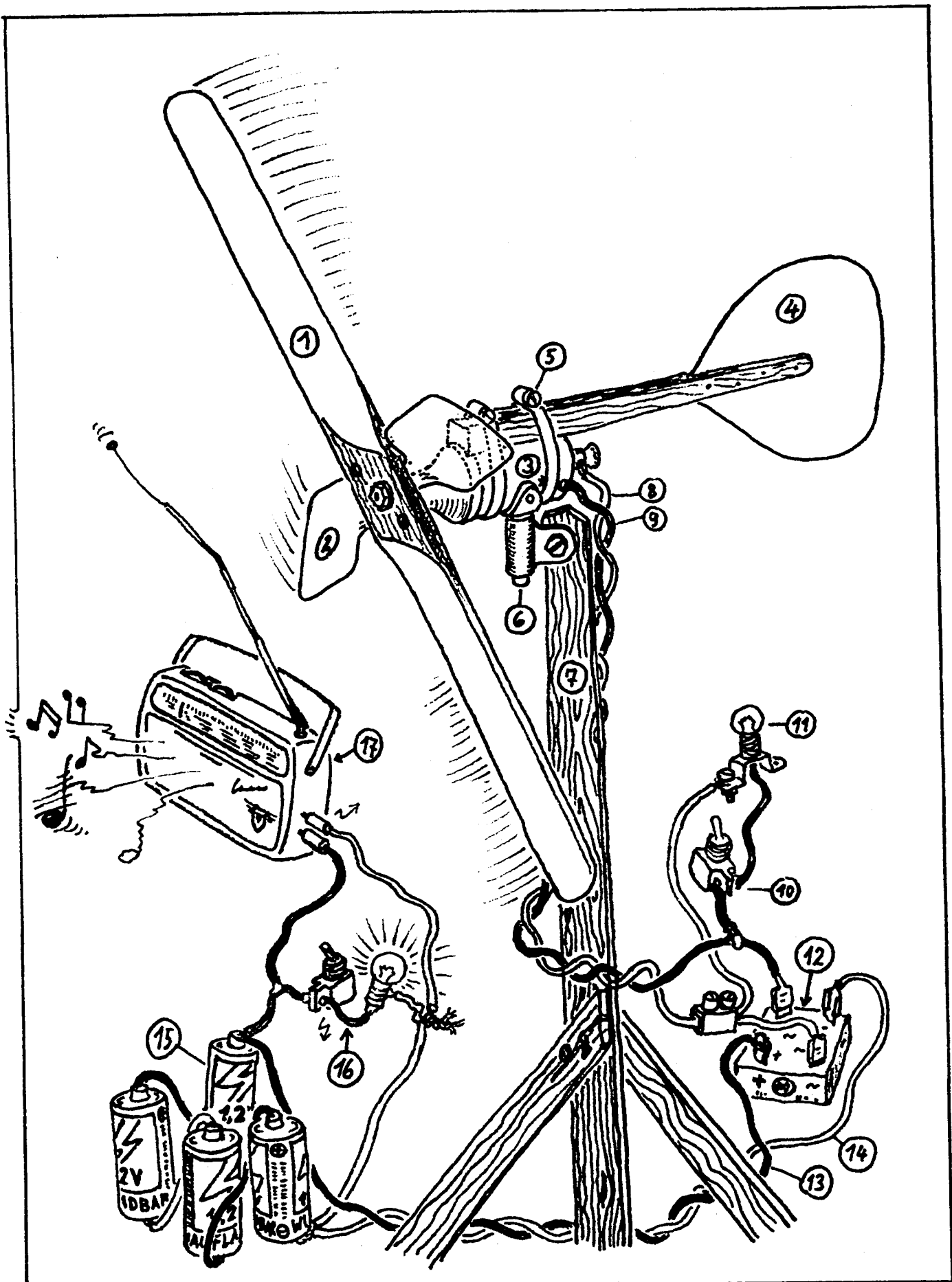
Einfachstes Windrad mit Fahrraddynamo, 50-cm-Repeller.
