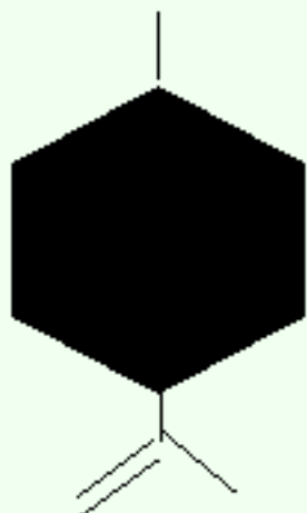
Limonene
