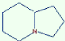
Indolizidine Nucleus
