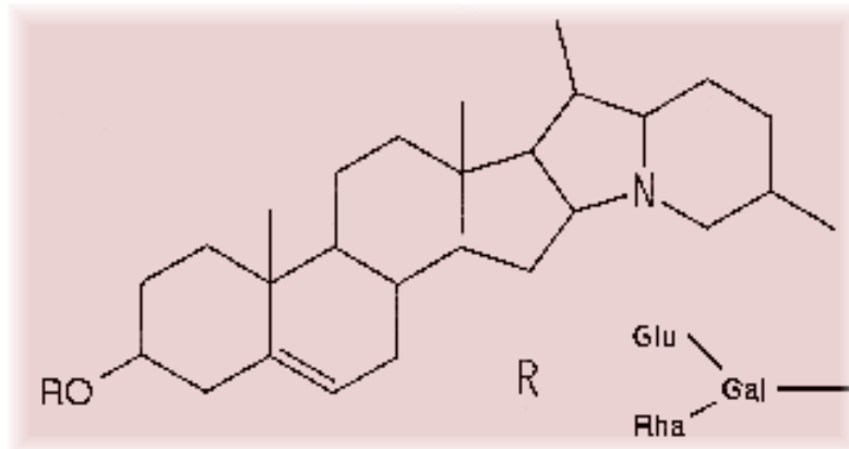
solasodine
