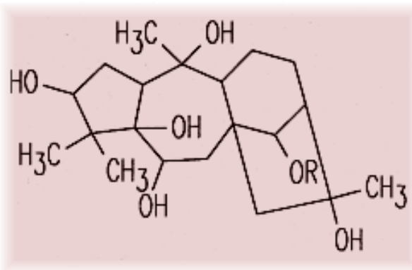
phytolaccigenin
