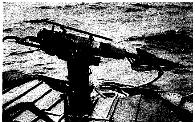
Fig 63 Whaling gun with pointed grenade. (Photo: Erste Deutsche Walfang Gesellschaft.)
