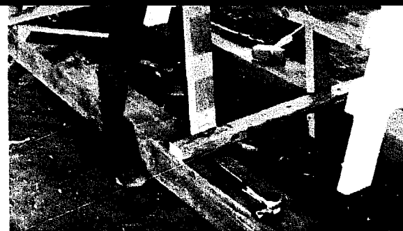
Fig.77 Installer les membrures à cheval sur les planches de montants de façon à ce que les traverses touchent la face des planches et que les côtés des membrures embarquent sur les côtés des planches. Les traverses doivent donner vers le centre de la pirogue. Vérifier que la traverse du bas de la membrure soit partout à l'égalité du dessus de la planche de montant
