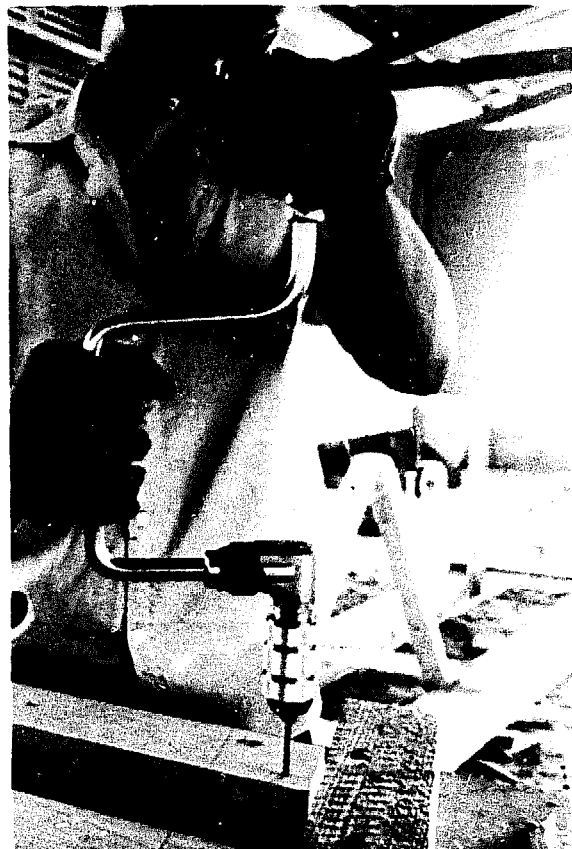
Fig.73 Percer les trous de 4 cm de profondeur avec un foret de 4 mm ou avec un clou dont la pointe a été aplatie à cette largeur. Laisser le foret dépasser de 4 cm du vilebrequin
