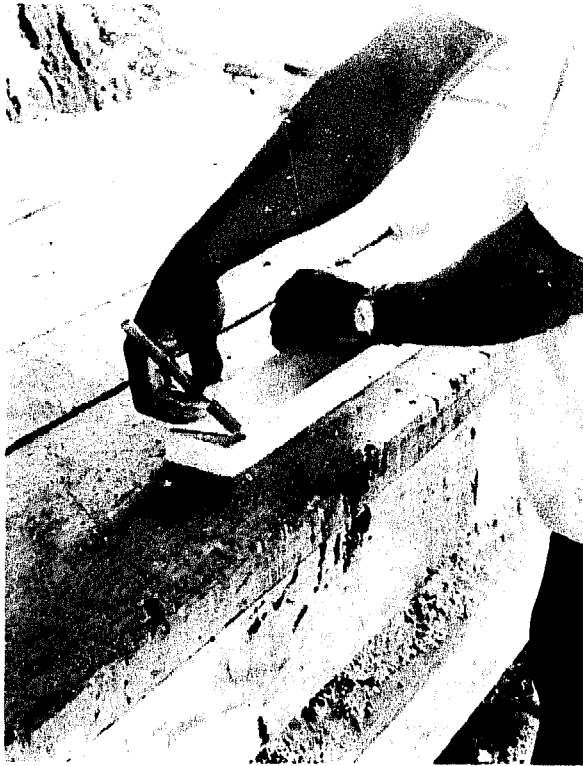
Fig.69 Tracer quatre côtés, C deux traverses du haut A et deux traverses du bas B avec les gabarits de traçage
