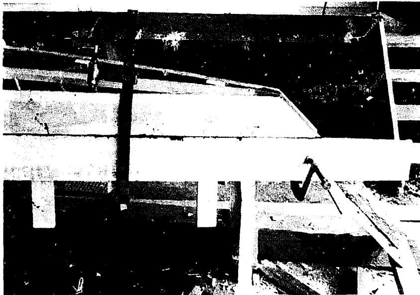
Fig.133 S'assurer qu'il y en a sur les côtés des étraves. Fixer à l'étrave comme pour le bouchain mais avec des clous de 7 cm
